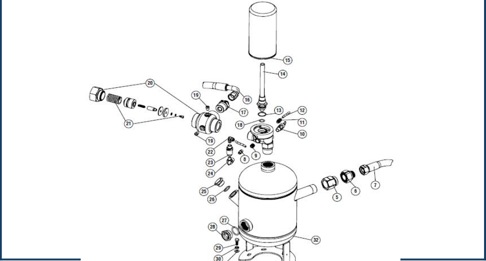
ITEM CODIGO | COD DESCRIÇÃO DECOMPOSICIÓN DECOMPOSITION QTD. | QTY 1 028-0751-QAT Manguera hidráulica - 700mm Manguera hidráulica - 700mm 700mm hydraulic hose 2 2 028-0351-QAT Manguera hidráulica - 750mm Manguera hidráulica - 750mm 750mm hydraulic hose 3 028-0520-QAT Manguera hidráulica - 630mm Manguera hidráulica - 630mm 630mm hydraulic hose 4 028-0448-QAR Manguera hidráulica - 560mm Manguera hidráulica - 560mm 560mm hydraulic hose 1
